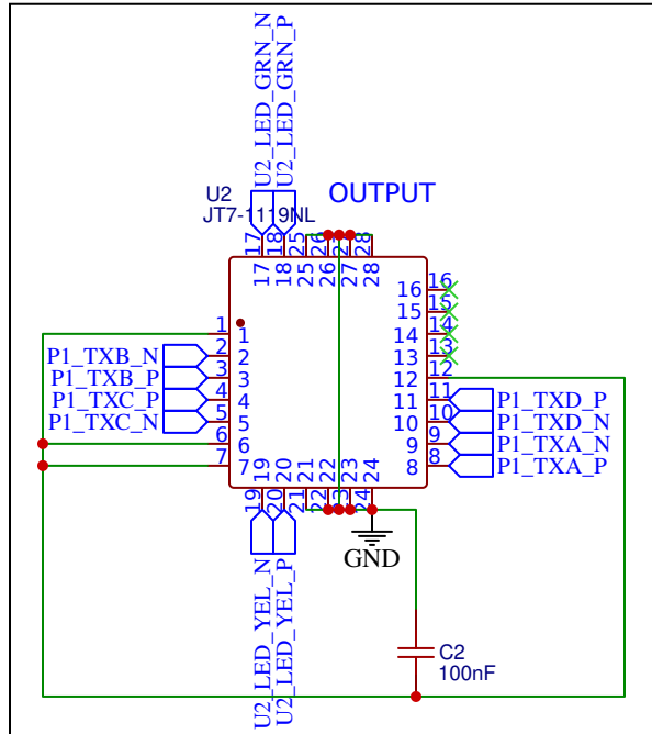
Ethernet Port (Output) - Jack
